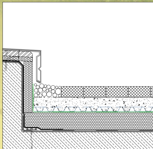
DELTA®-FLORAXX – využitá plochá strecha s dlažbou, obrátená skladba, oplechovaná atika.
