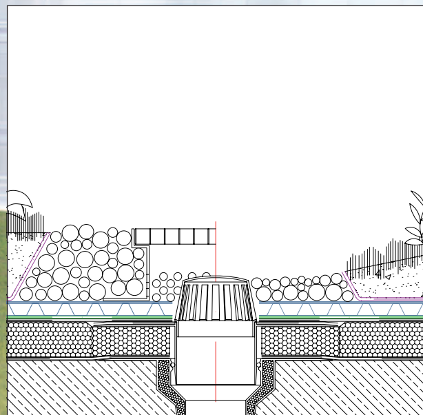
DELTA®-FLORAXX TOP – napojenie na strešný vpust.
